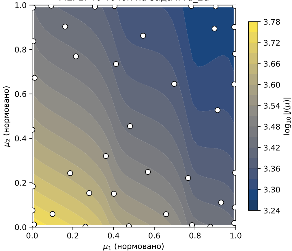
МЕРЕ: 40 точок на задачі rd_2d
